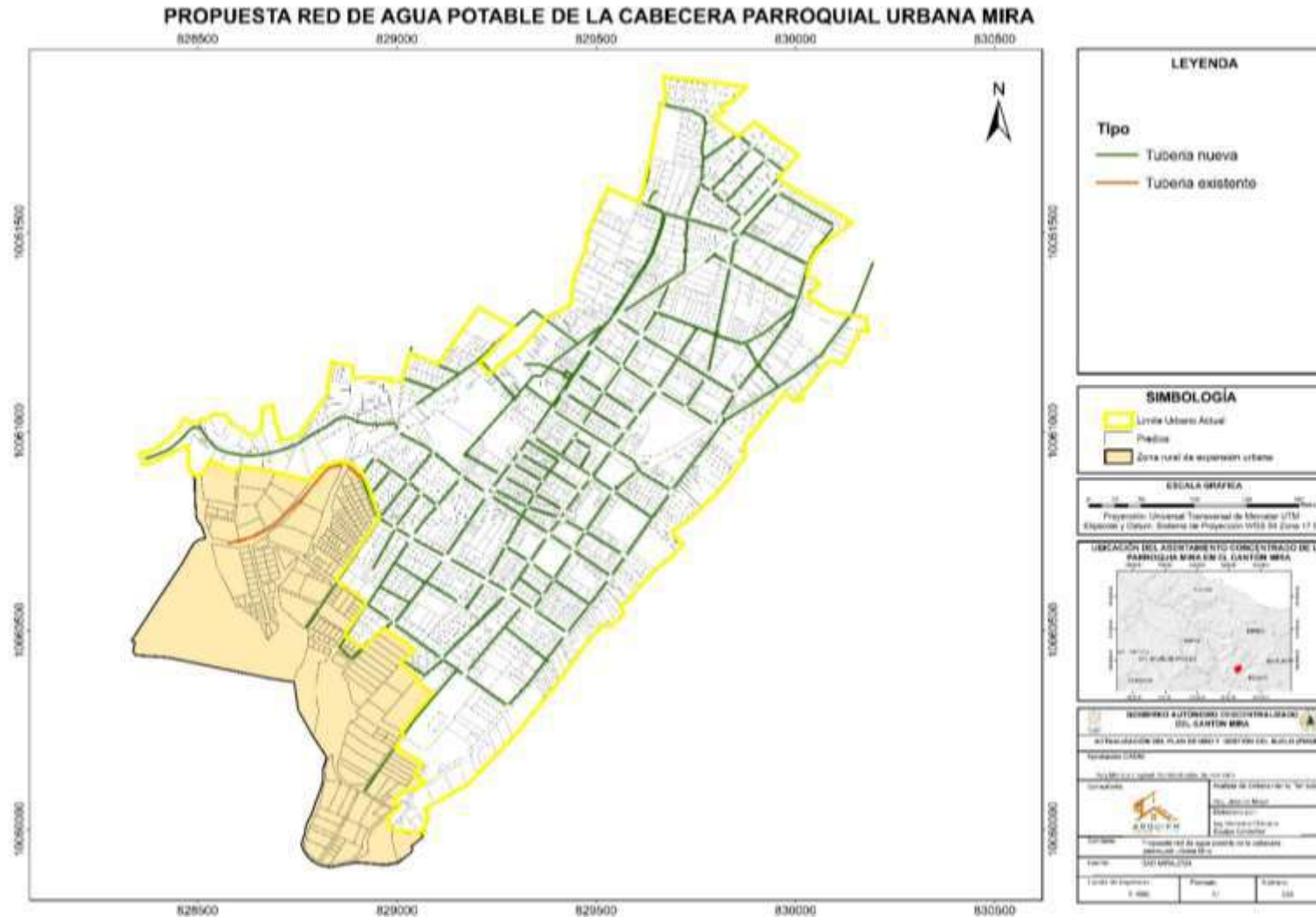
MAPA 69. Propuesta de Red de agua potable cabecera parroquial Mira.
