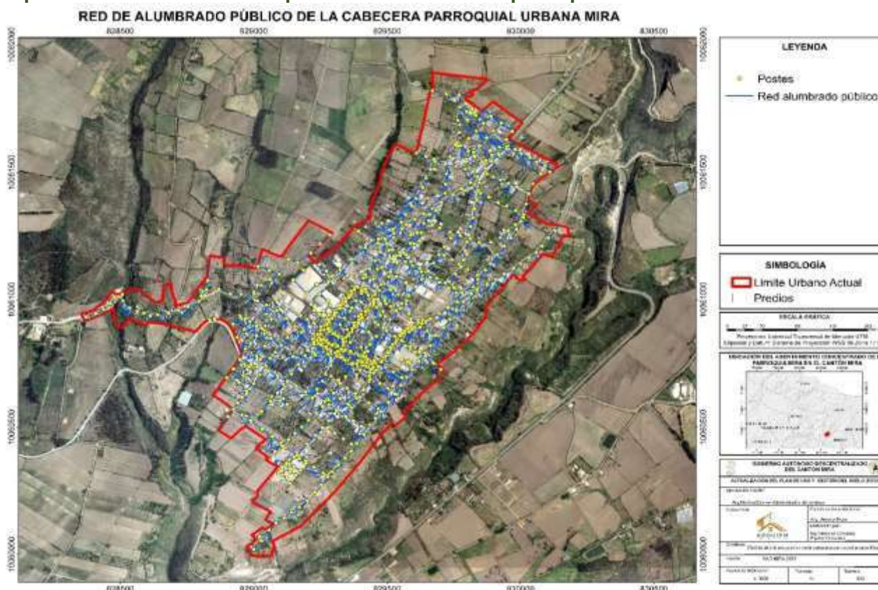
Mapa 31. Red de alumbrado público de la cabecera parroquial urbana Mira.
