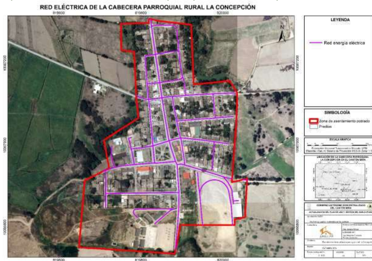
Mapa 22. Red eléctrica de la cabecera parroquial rural La Concepción.
