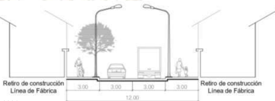
Tipología de vía Local A
