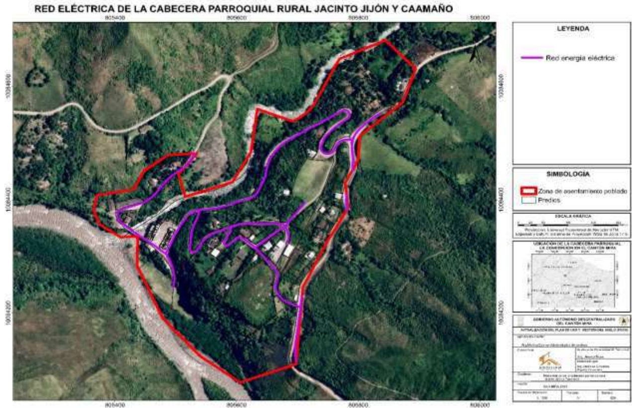
Mapa 27. Red eléctrica de la cabecera parroquial rural Jacinto Jijón y Caamaño
