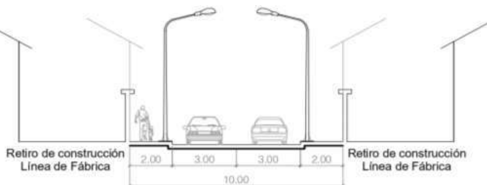
Tipología de vía Local B
