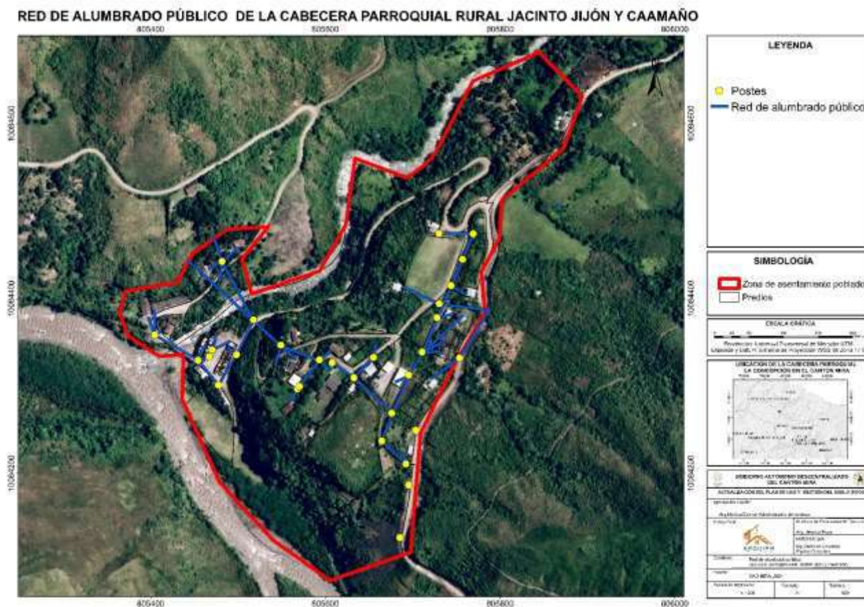
Mapa 26. Red de alumbrado público de la cabecera parroquial rural Jacinto Jijón y Caamaño
