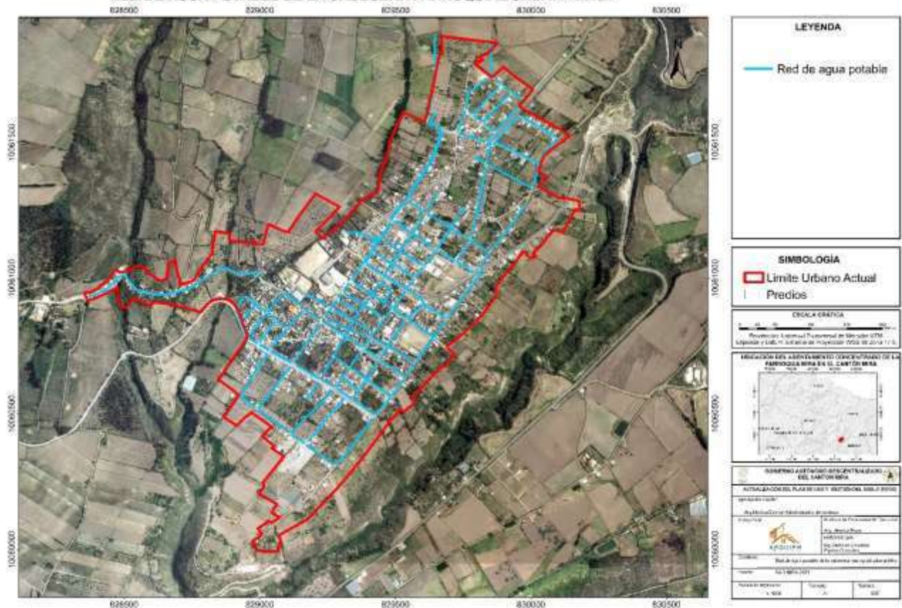
RED DE AGUA POTABLE DE LA CABECERA PARROQUIAL URBANA MIRA
