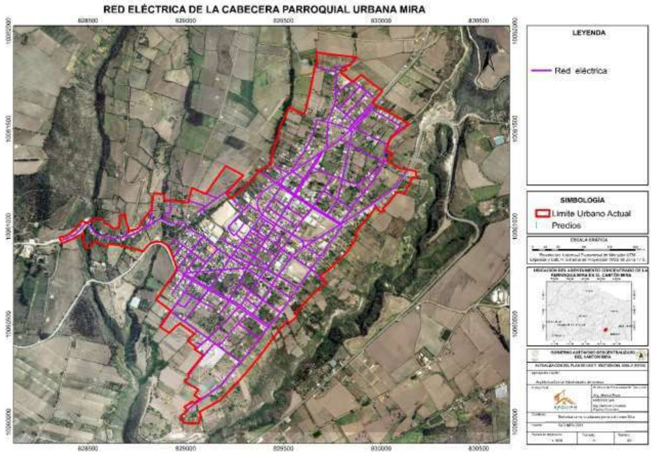
Mapa 32. Red de energía eléctrica de la cabecera parroquial urbana Mira
